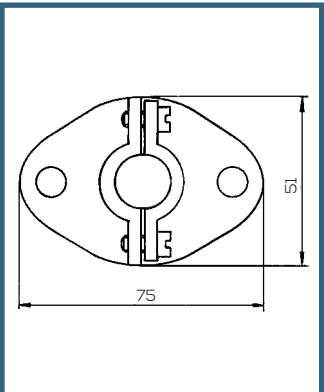
FLANGE
